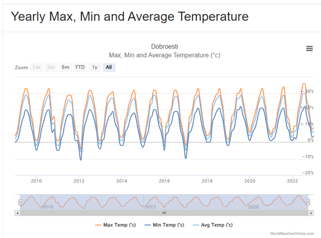
Figură 13 – Evoluția temperaturilor pe ultimii 12 ani
